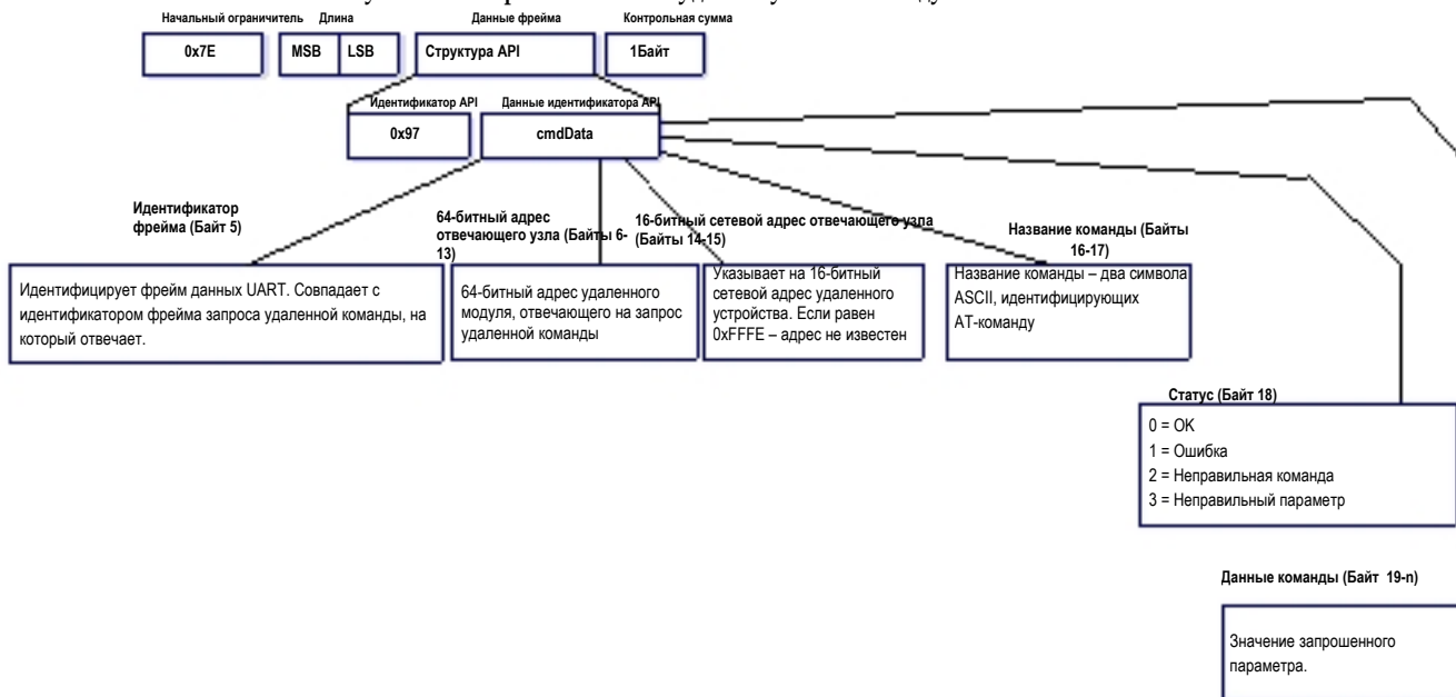
Рисунок 7-12. Фрейм ответа на удаленную AT-команду.
