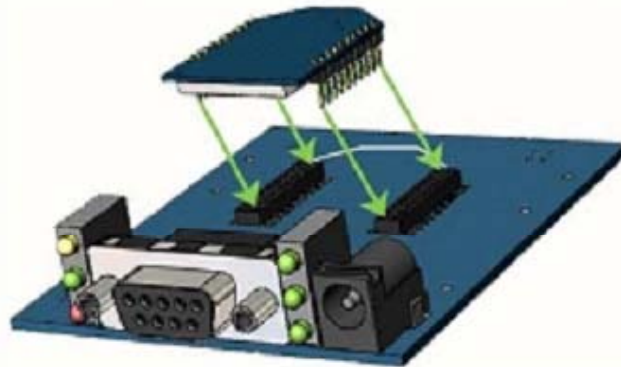
Рисунок 1-02. Установка модуля XBee Series 2 на плату с интерфейсом RS-232.
