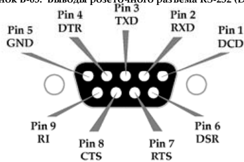
Рисунок В-03. Выводы розеточного разъема RS-232 (DB-9) последовательного порта
