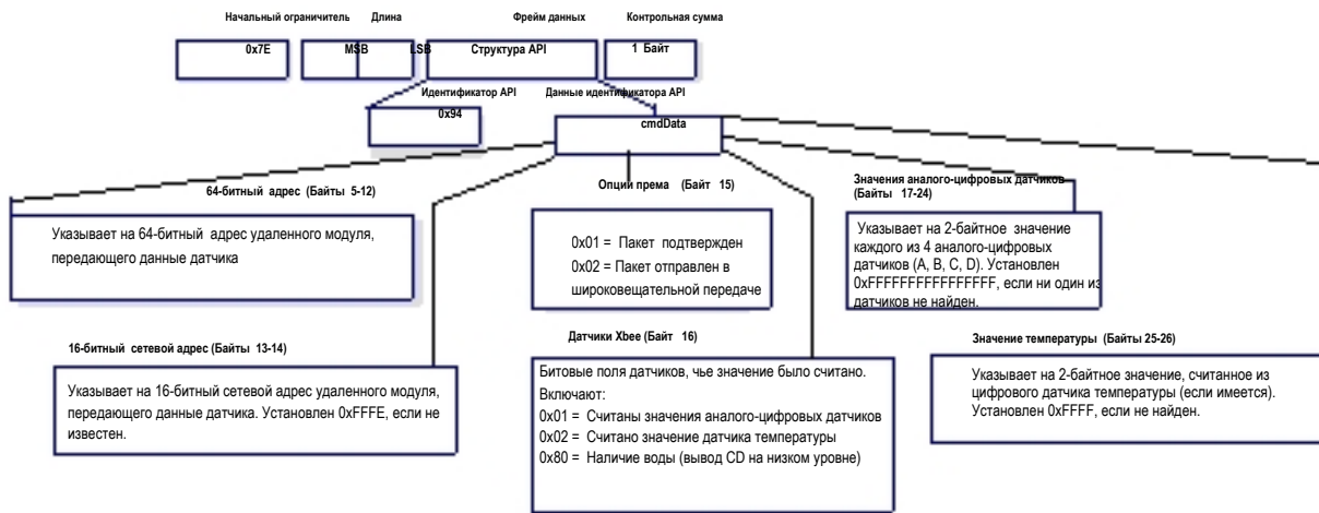
Рисунок 7-18. Фрейм индикатора чтения датчика (0x94)
