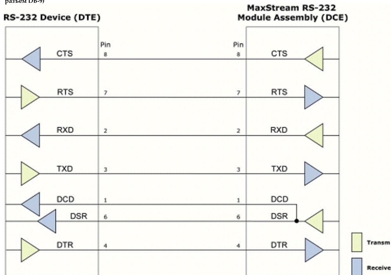
Рисунок В-04. Узел DTE (RS-232, вилочный разъем разъема DB-9), соединенный с модульной сборкой DCE (розеточный разъем DB-9)
