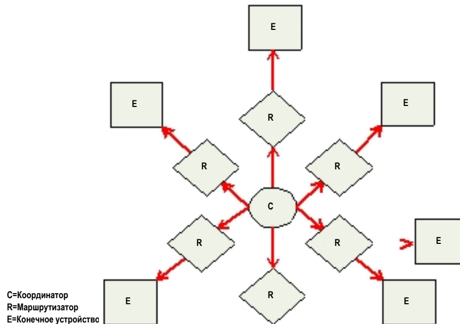
Рисунок 3-04. Передача данных в широковещательном режиме
