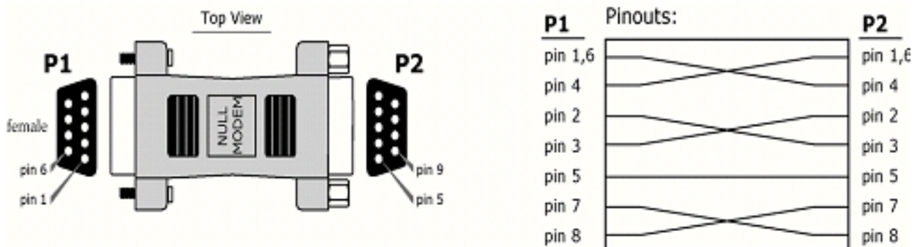
Рисунок В-09. Розеточный разъем и выводы нуль-модемного адаптера
