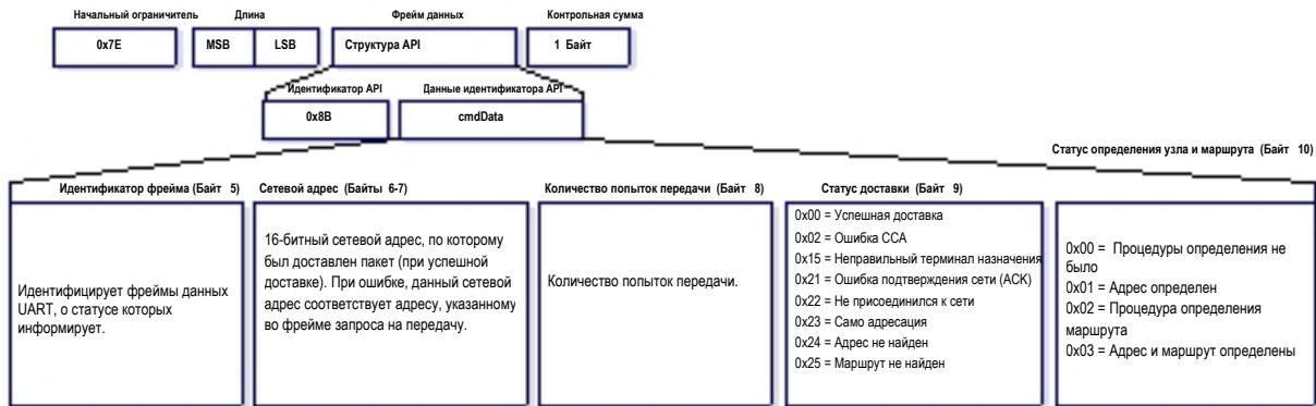
Рисунок 7-15. Фрейм статуса передачи
