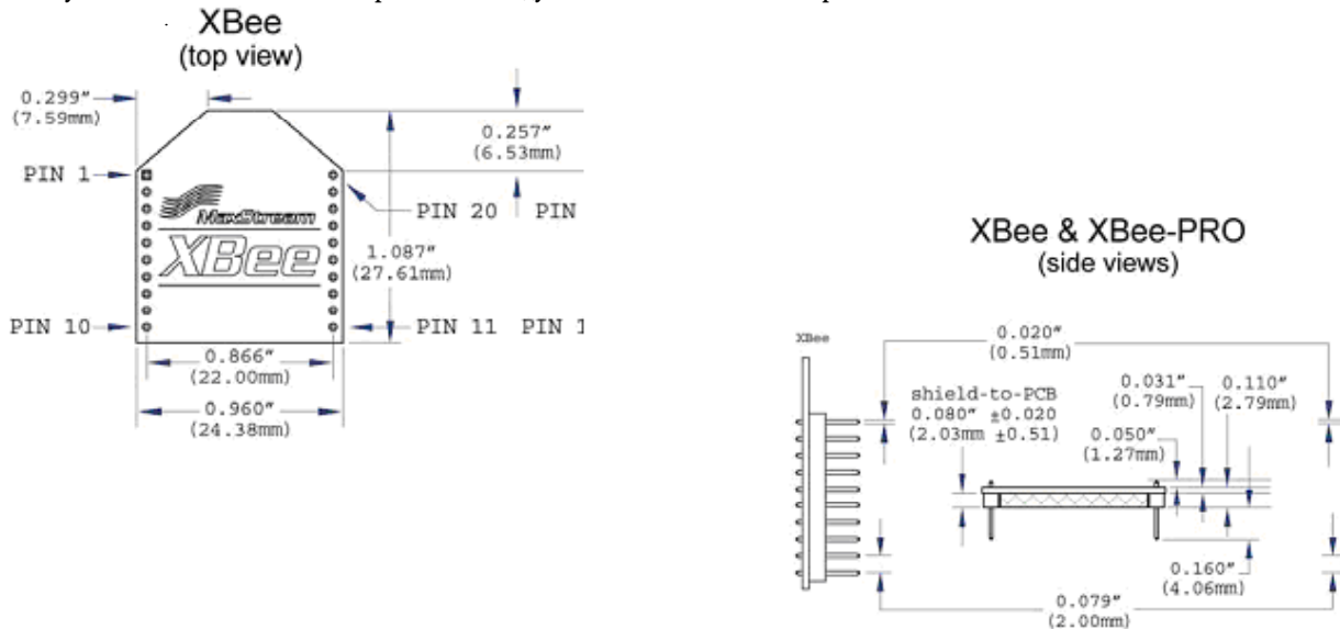
Рисунок 1-01. Механические чертежи RF-модулей XBee Series 2 OEM (варианты антенн не показаны)
