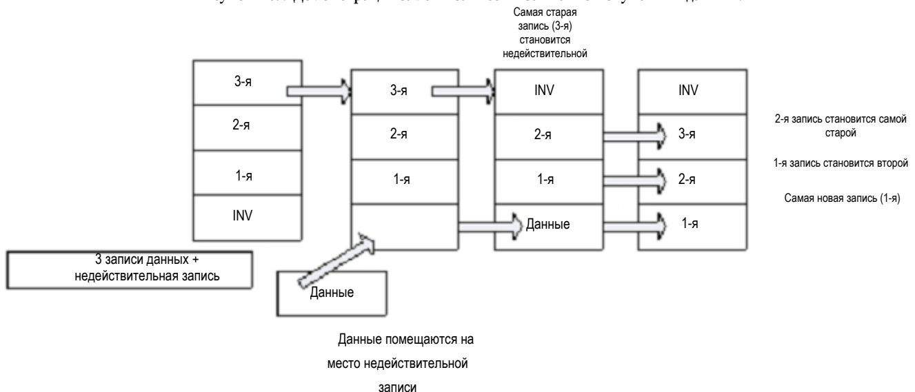
Рисунок 4-09. Демонстрация замены записей в Записях о полученных данных.
