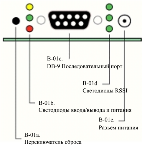
Рисунок В-01. Вид спереди
