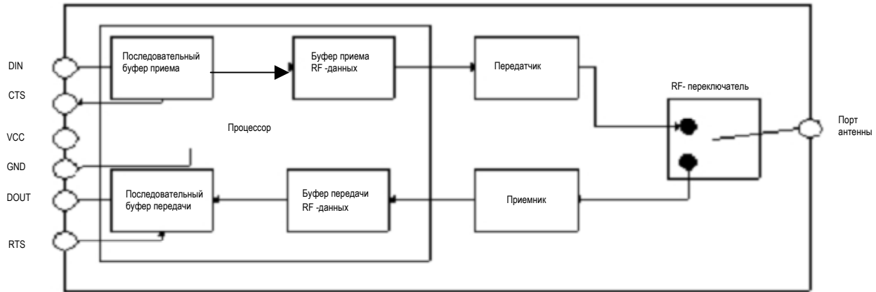
Рисунок 2-03. Диаграмма внутреннего обмена данными
