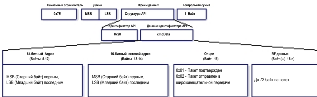
Рисунок 7-16. Фрейм приема пакета
