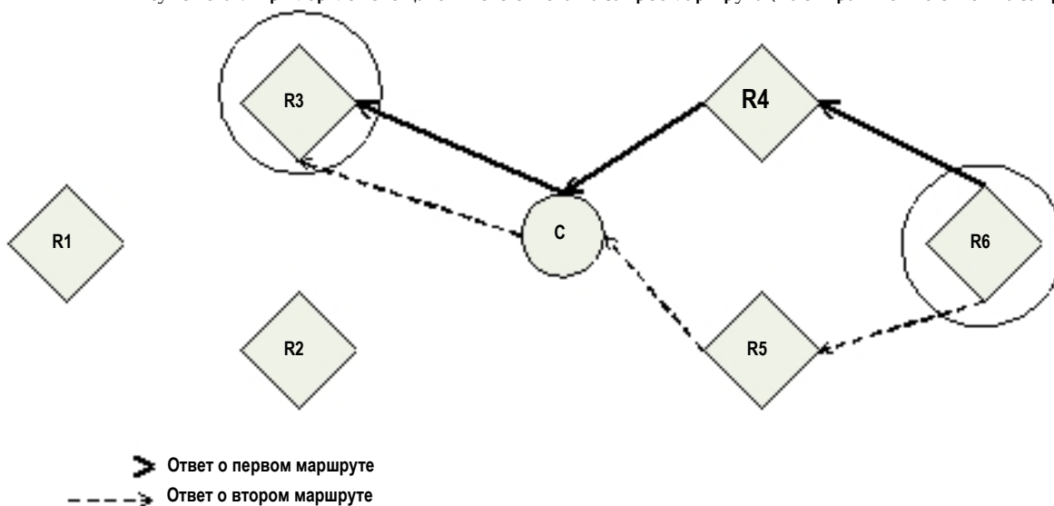
Рисунок 3-07. Пример моновещательного ответа на запрос маршрута (R6 отправляет R3 ответ на запрос маршрута)
