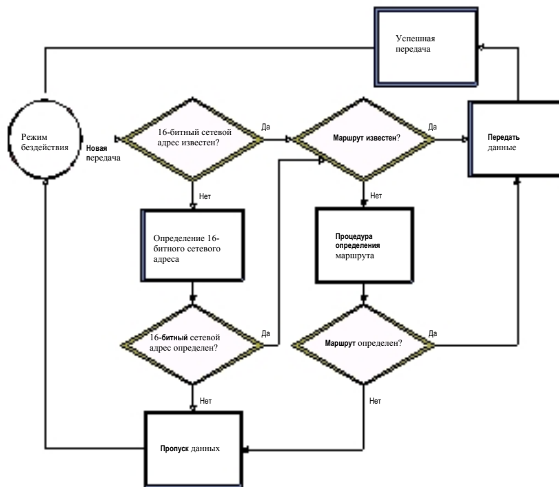
Рисунок 2-04. Последовательность Режимы передачи
