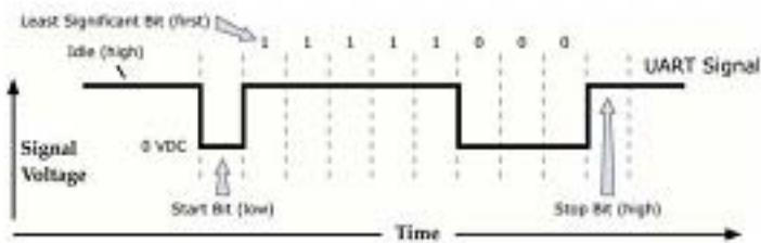
Рисунок 2-02. Пакет данных UART 0x1F (десятичное число "31") в момент передачи в RF-модуль. Пример формата данных 8-N-1 (биты - парность - #бит остановки)
