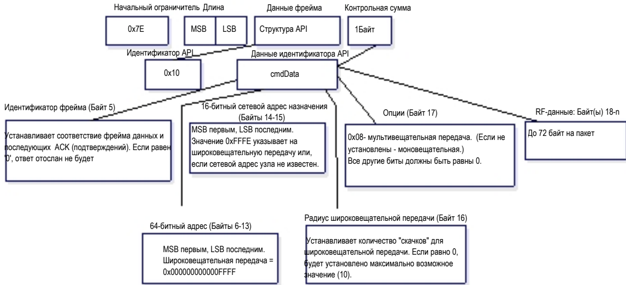
Рисунок 7-13. Запрос на передачу ZigBee.
