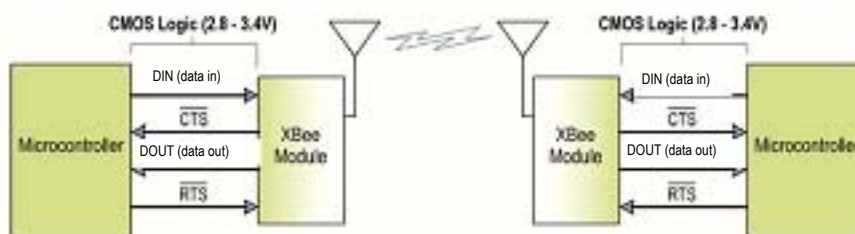
Рисунок 2-01. Диаграмма системного обмена данными через интерфейс UART (Сигналы с управлением по нижнему уровню показаны с горизонтальной полосой над названием)
