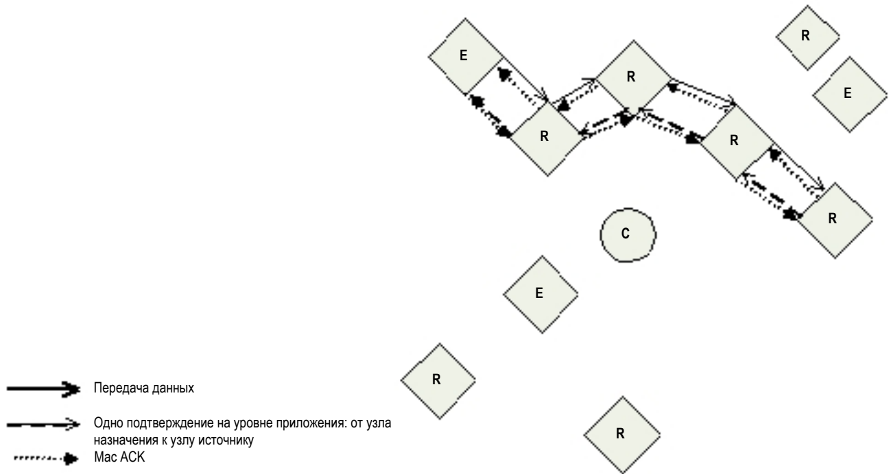
Рисунок 3-08. Монобещательная передача данных
