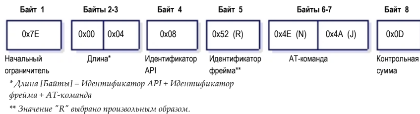
Рисунок 7-8. Пример: Фреймы API для изменения параметра NJ модуля.
