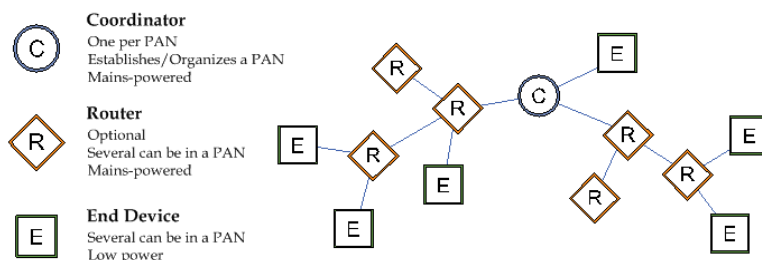
Рисунок 3-01. Типы узлов / Пример простой топологии сети ZigBee
