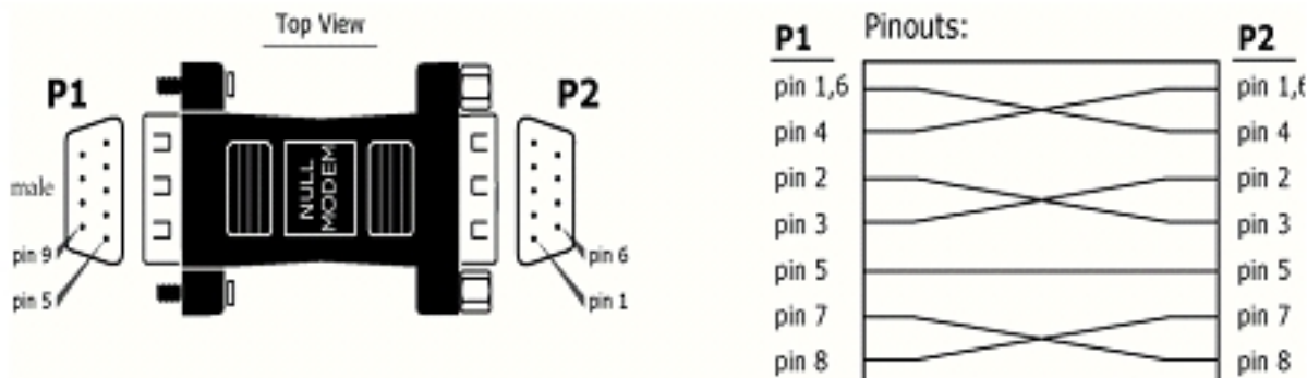
Рисунок В-07. Вилочный разъем и выводы нуль-модемного адаптера
