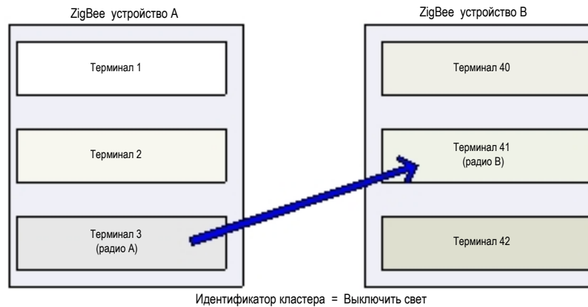
Рисунок 3-03. Пример адресации на уровне приложений
