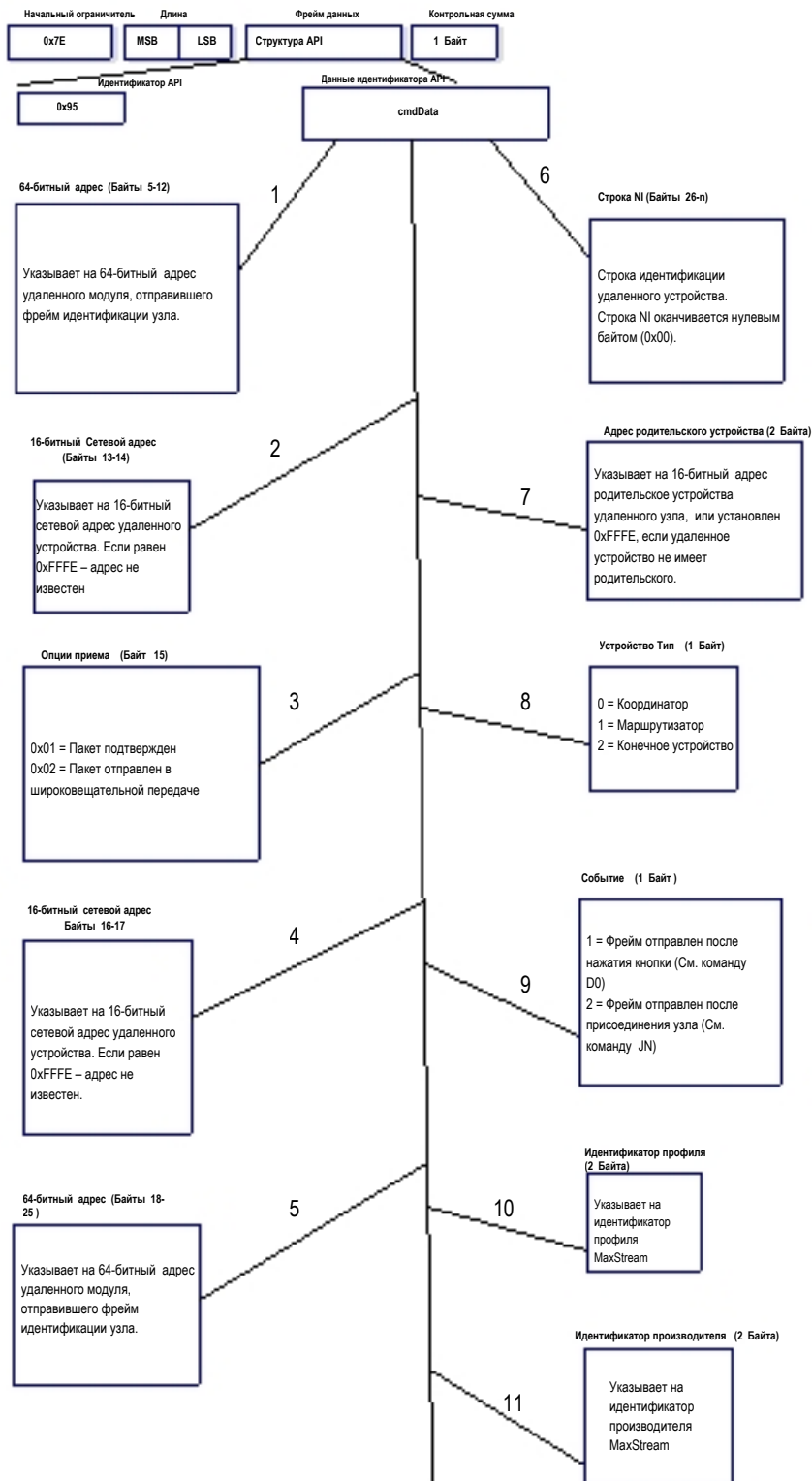
Рисунок 7-19. Фрейм идентификации узла
