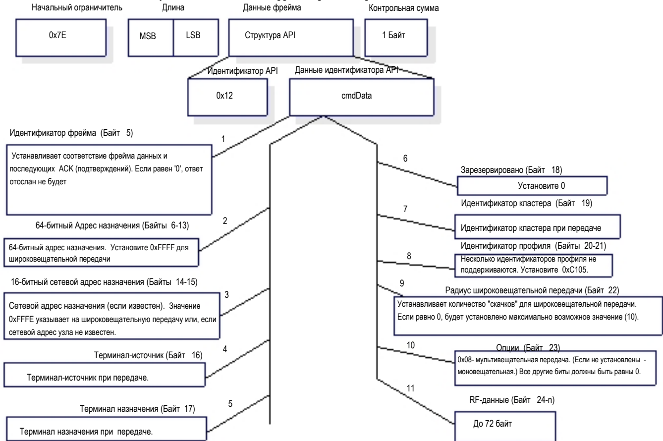
Рисунок 7-14. Командный фрейм прямой передачи
