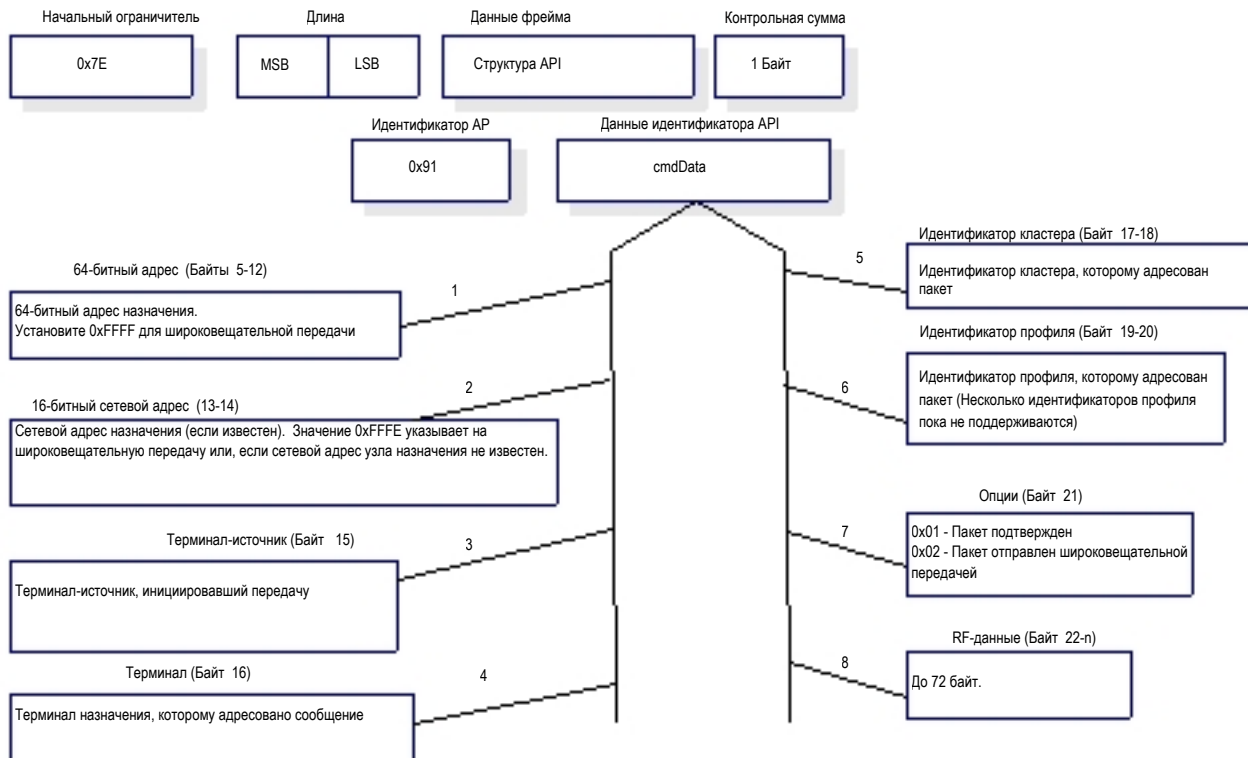
Рисунок 7-17. Индикаторы прямого приема ZigBee
