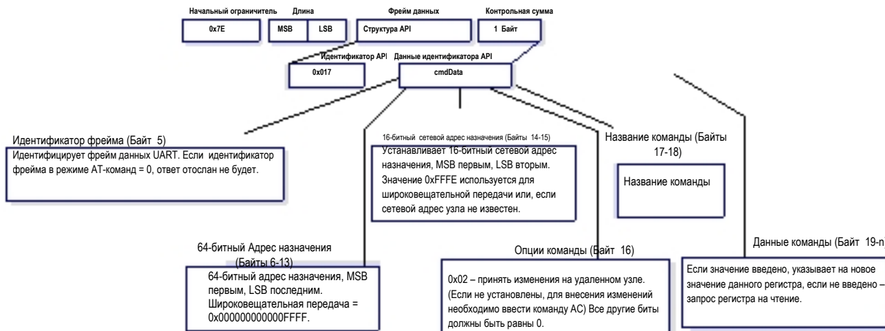
Рисунок 7-11. Фрейм запроса удаленной команды
