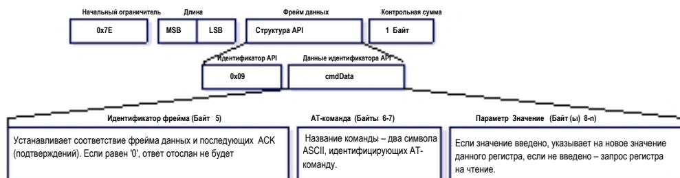
Рисунок 7-9. Фрейм AT-команд с очередью параметров (фрейм идентичен фрейму AT-команд, за исключением идентификатора API.)
