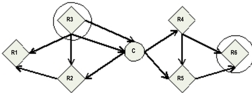
Рисунок 3-06. Пример широковещательного запроса маршрута (R3 пытается определить маршрут к R6)
