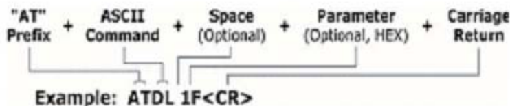
Рисунок D-05. Синтаксис AT-команд
