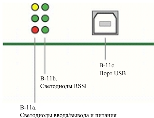
Рисунок D-02. Вид спереди
