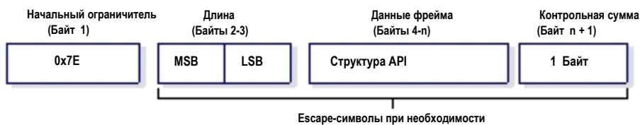
Рисунок 7-02. Структура UART фреймов данных с управляющими escape-символами:
