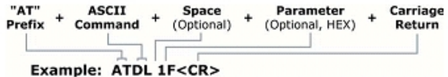
Рисунок 2-05. Синтаксис АТ-команды
