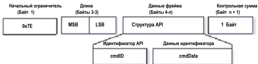
Рисунок 7-03. UART фрейм данных и структура API-данных:
