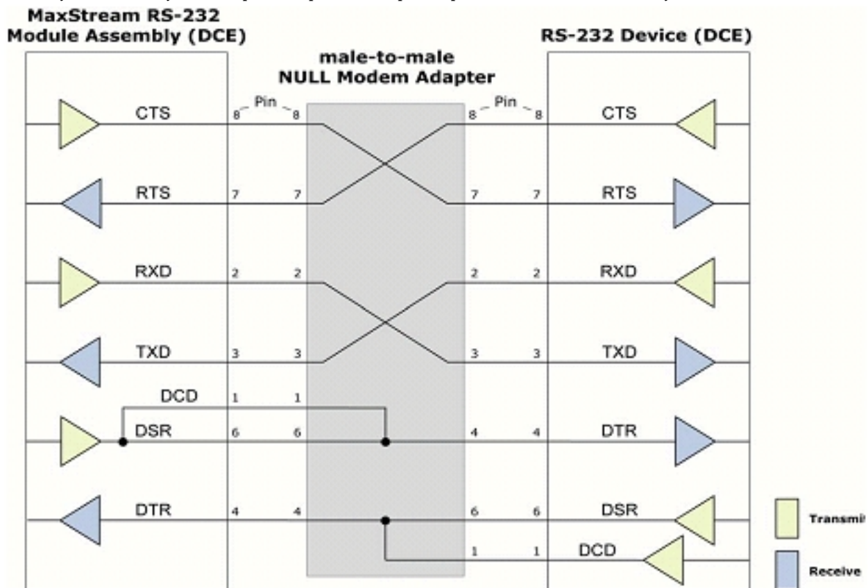
Рисунок В-05. Модульная сборка DCE (розеточный разъем DB-9), соединенный с узлом DCE (RS-232, вилочный разъем DB-9)
