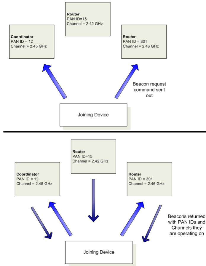
Рисунок 3-02. Демонстрация обмена сообщениями (Beacons) при присоединении устройств
