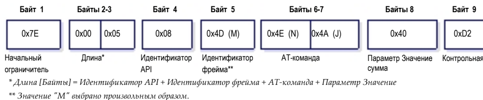
Рисунок 7-8. Пример: Фреймы API для изменения параметра NJ модуля.
