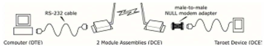
Рисунок В-06. Типовая беспроводная связь между узлами DTE и DCE
